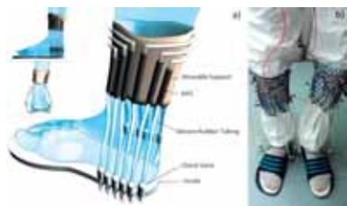
Bản vẽ thiết kế (a) và hình ảnh sản phẩm thực (b). Ảnh: MIT
